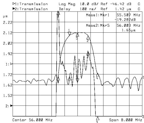
Horizontal: 0.8MHz/Div Vertical: 100ns/Div&10dB/Div
